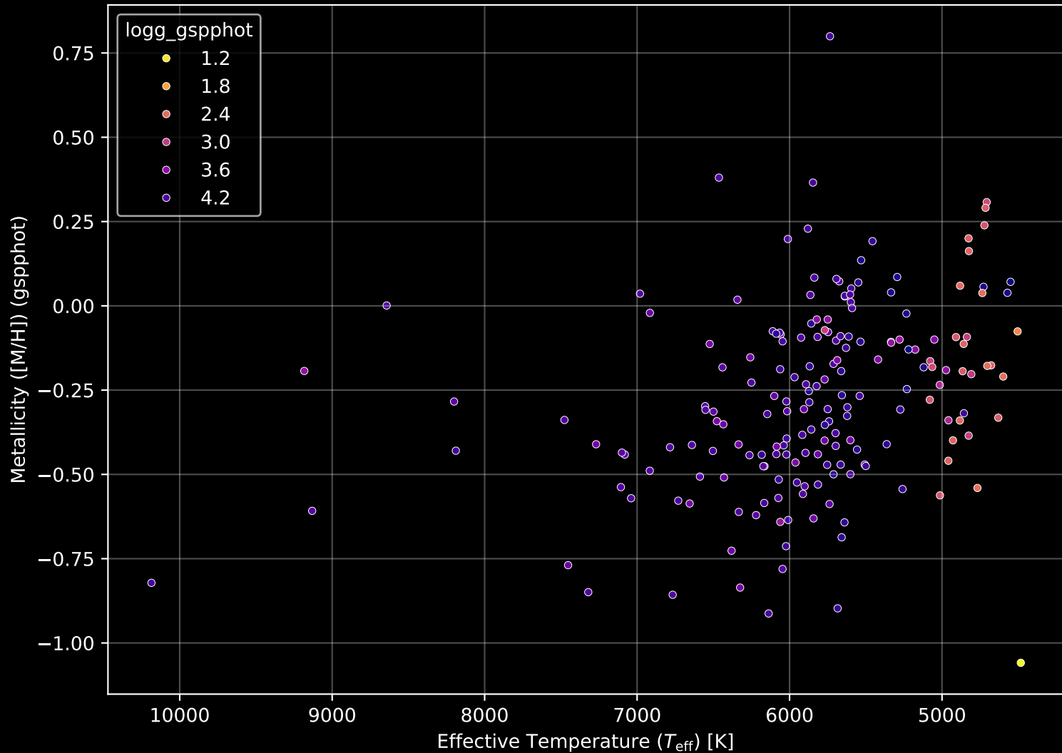
GALAH DR4 Field: [7130] Stellar Population Parameters (n= 189)
