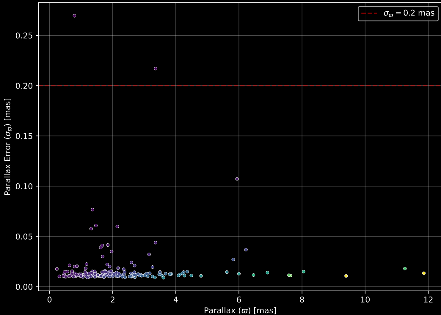
GALAH DR4 Field: [7130] Parallax Quality (n= 189)
