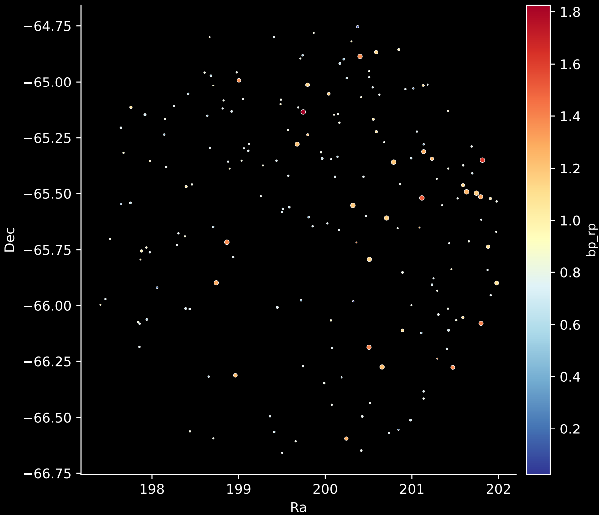
GALAH DR4 Field: [7130] Stars: 189
